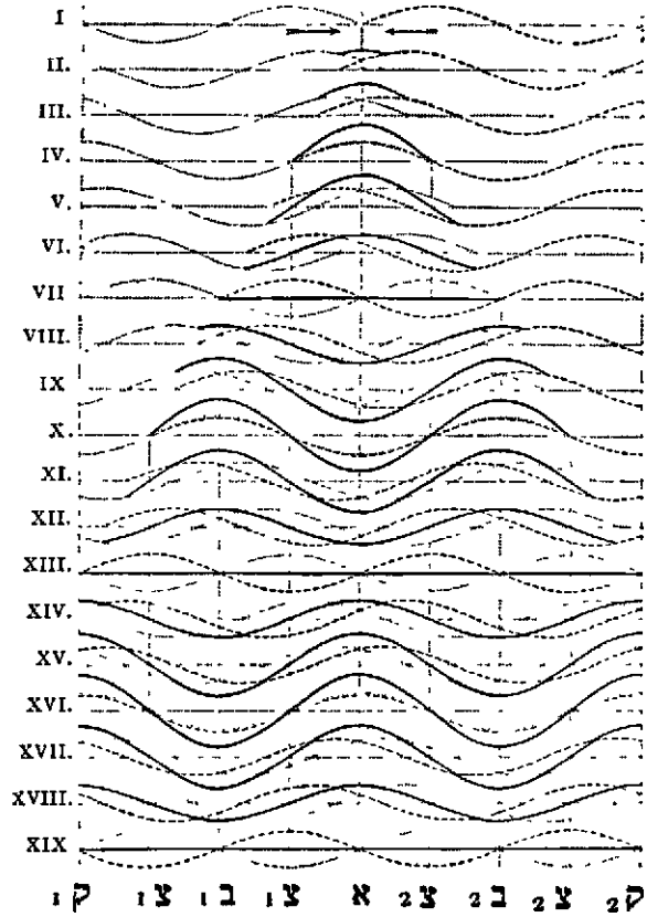
ציור 6 התהוות גל עומד ספגש בין שני גלים שווים-מדרגת, המתפשטים בכיוונים נגדיים א, ב, ג — נקודות-בטן ד, ה — נקודות-צומת ו, ז — קצוות
